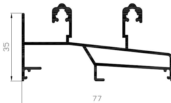
Marco fijo c.clip Ref: 8211
