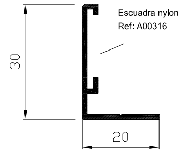
Solape 30 mm cajon compacto Ref: 9332
