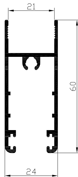
Hoja ruedas H=21 mm Ref: 9234
