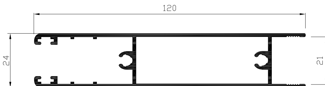
Zócalo H=21 mm Ref: 9237
