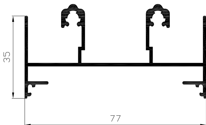
Marco fijo sin clip Ref: 8212
