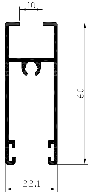
Hoja ruedas H=10 mm Ref: 9204
